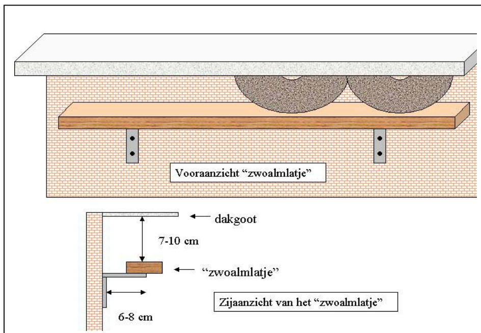
Fig. 22: Voor- en zijaanzicht van het “zwoalmlatje”
